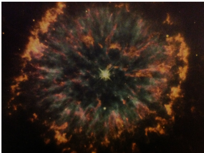
Foto van een supernova, een grote exploderende ster. Volgens Rudolf Steiner hangt zo'n explosie samen met de incarnatie van een grote individualiteit op de aarde.
